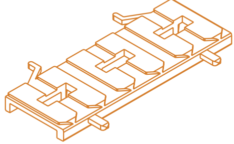
Cam Takožu Glass Wedge (Thick) Подкладка стеклопакета تسميكة الزجاج
